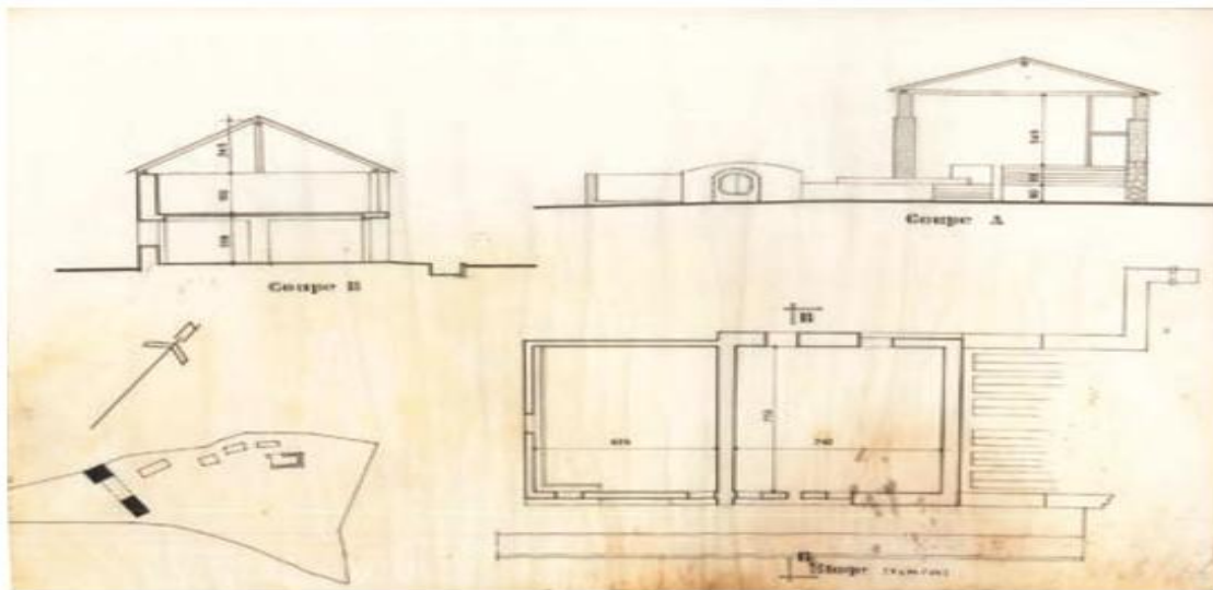
Profil des bâtiments A et B de la distillerie Fond-Rousseau, 1985
